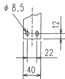
導帯本体 じか付 端子寸法
