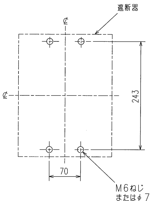
穴明寸法
