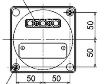
取付ねじ M5
